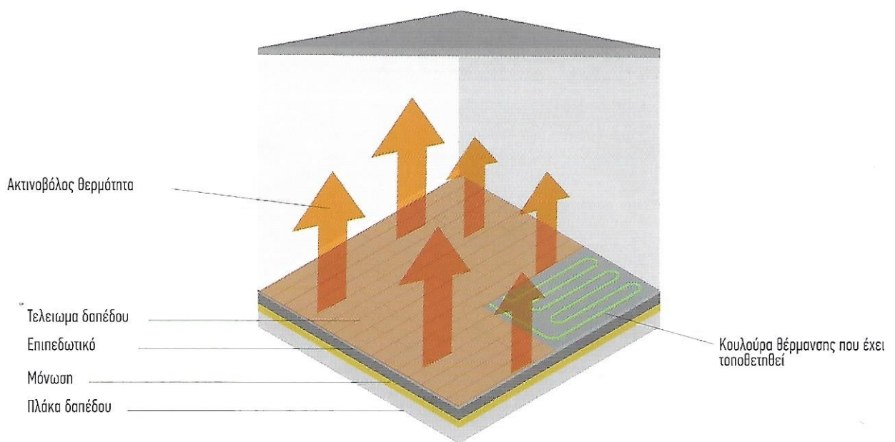
Μετάδοση θερμότητας: Ενδοδαπέδια θέρμανση
